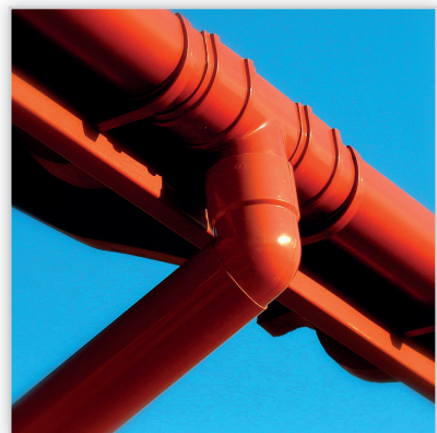
LEMAR, Systemy rynnowe. Materiał: nieplastifikowany PVC-U (gr. 2 mm), rynna półokrągła, rura okrągła. Sr. rynny/rury spustowej [mm]: 150, 120, 85/110, 90, 75, 50. Dł. rynny/rury spustowej [m]: 6-2/6-0,5. Maks. pow. odwadniana (rura skrajnie/gustawie) [m²]: 180/370. Kolory: brąz, czerwony, biały, zielony. Normy: PN EN 607:2005, PN EN 12200-1:2002, EN 1462. Elementy systemu: haki, złączki leje spustowe, denka, rewizje, uchwyty, redukcje, narożniki, uszczelki gumowe.
